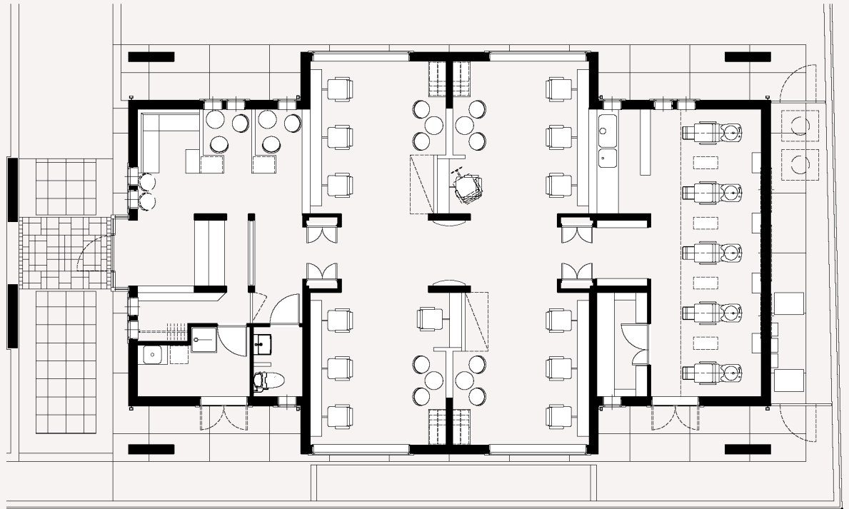
平面図
