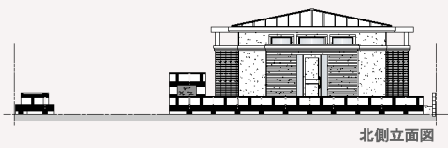
北側立面図
